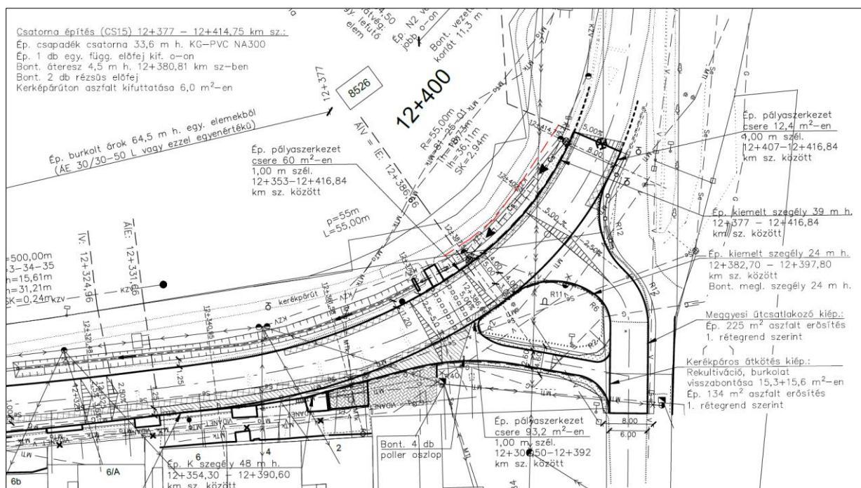
Helyszínrajz (piros szaggatott vonal: kisajátítási határ; készítette: Pannonway Kft.)
